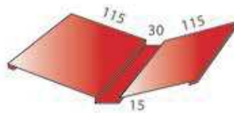
Ендова фигурная
