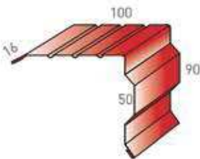
Планка торцевая фигурная
