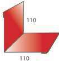
Планка угла внутреннего
