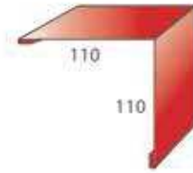
Планка угла внешнего
