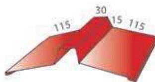
Конек плоский (фигурный)
